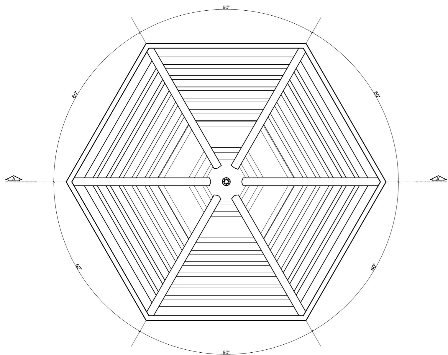
PLANTA BAIXA - PERGOLADO SALVA BRAVA esc 1:20
