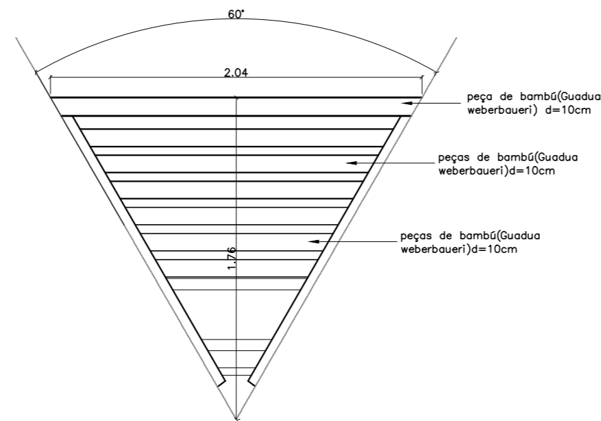
DETALHE esc 1:20
