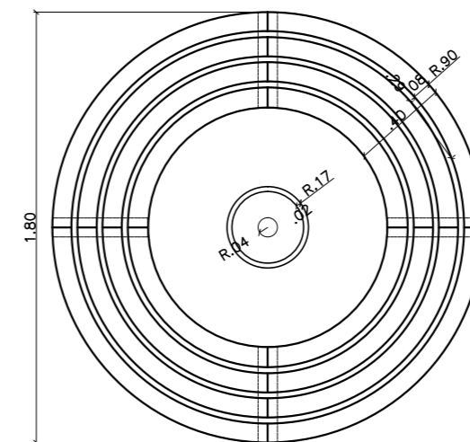
PLANTA BAIXA - BANCO/FLOREIRA CIRCULAR esc 1:20
