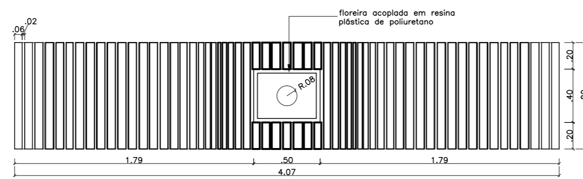
PLANTA BAIXA - ESPREGUIÇADEIRA/ FLOREIRA ACOPLADA esc 1:20
