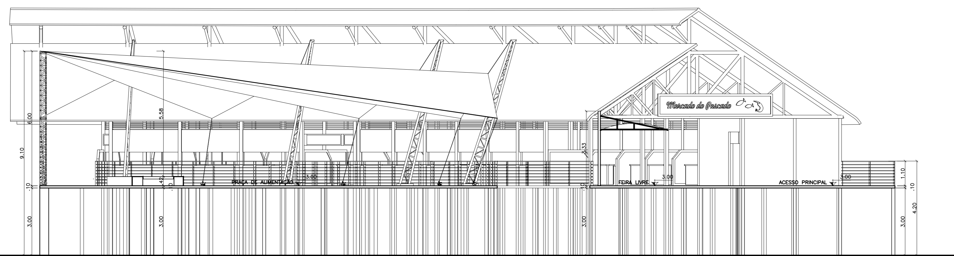
CORTE B esc. 1:100
