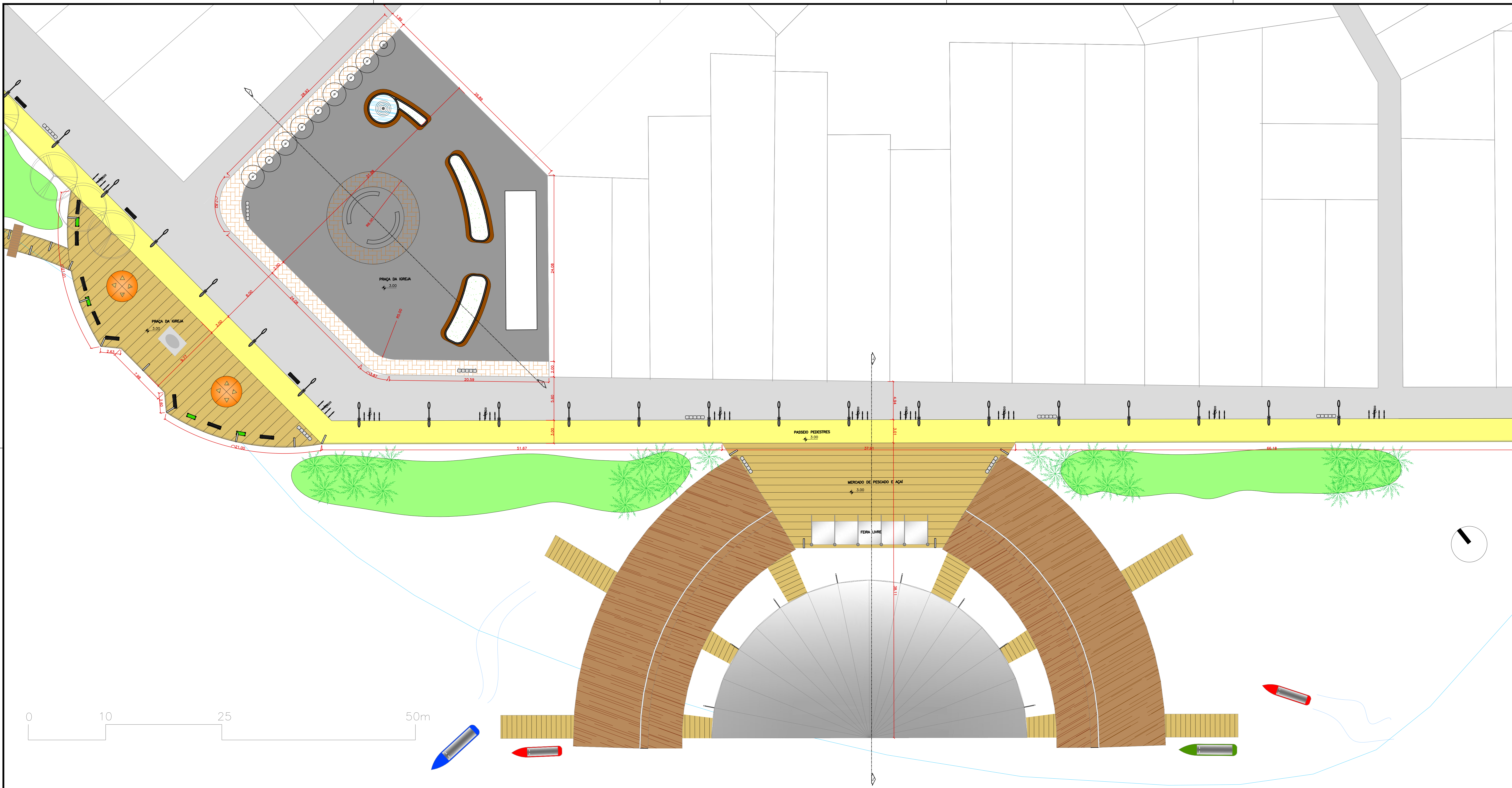
PLANTA BAIXA - EIXO 4 A 5 esc 1:200
