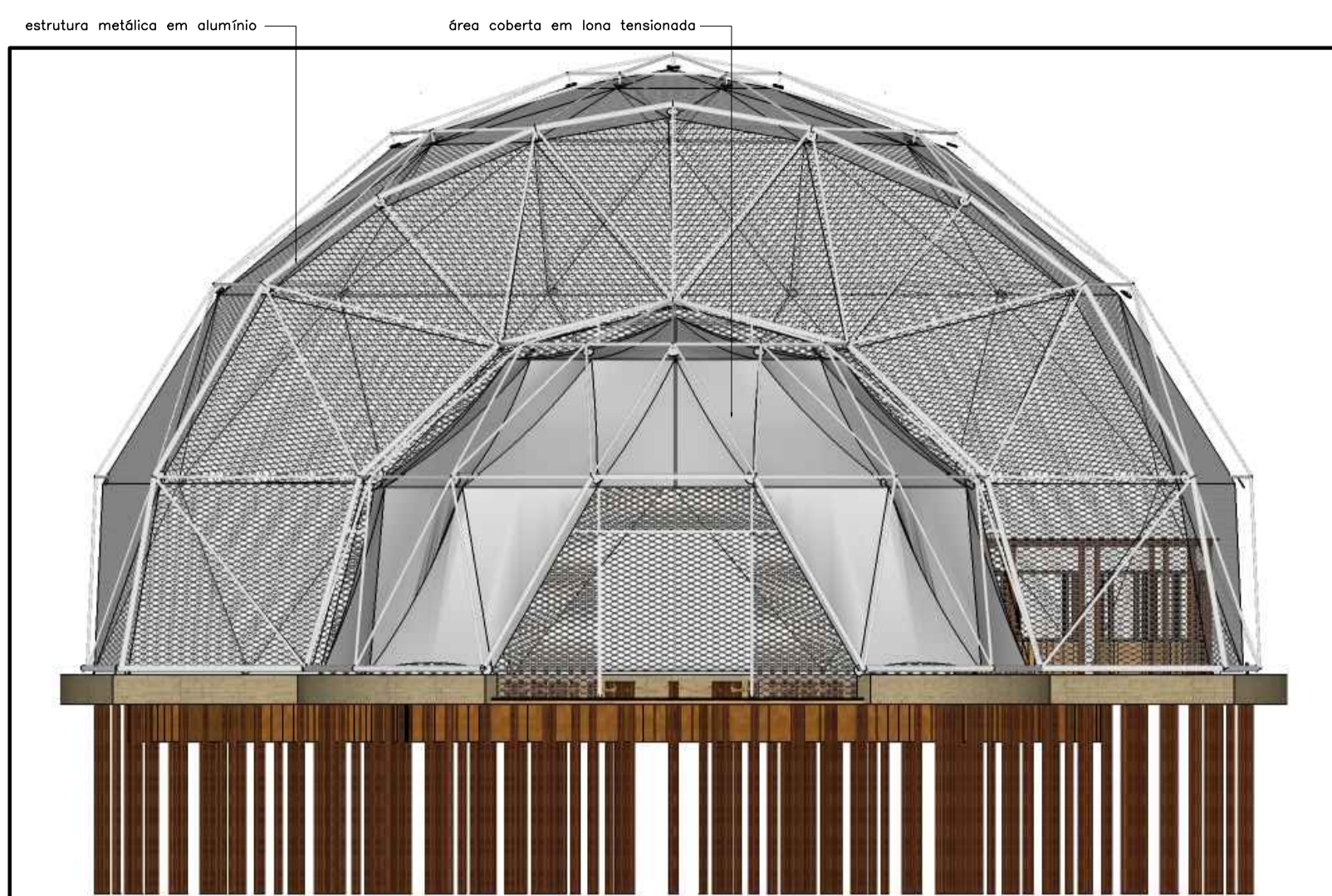
FACHADA FRONTAL esc 1:100
