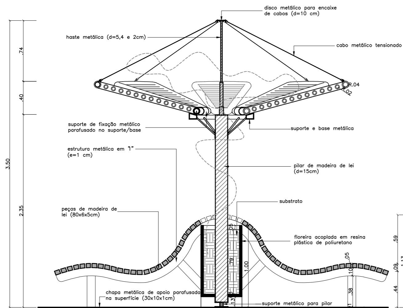
CORTE AA'- PERGOLADO / ESPREGUIÇADEIRA esc 1:20
