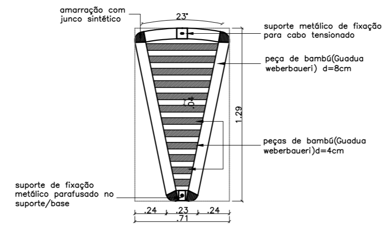
DETALHE - PÉRGOLA esc 1:20
