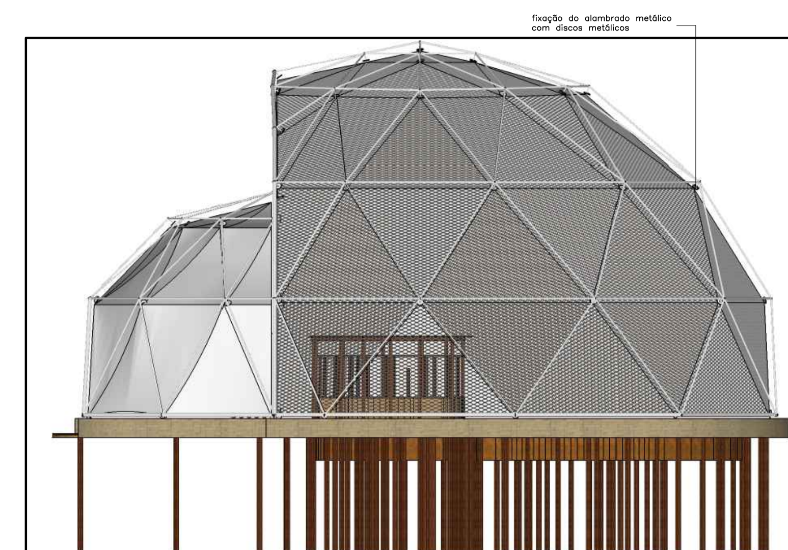
FACHADA FRONTAL esc 1:100
