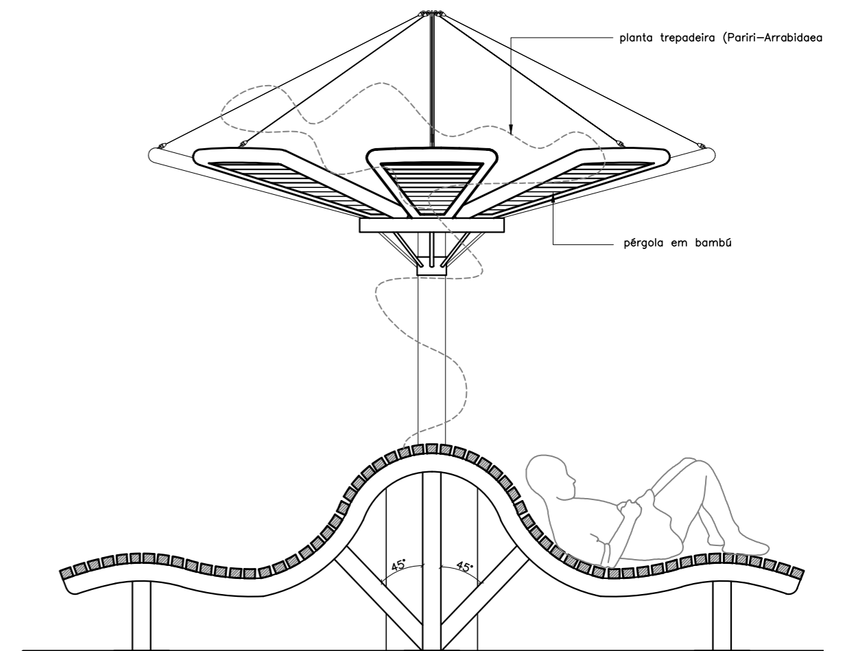
ELEVAÇÃO - PERGOLADO / ESPREGUIÇADEIRA esc 1:20
