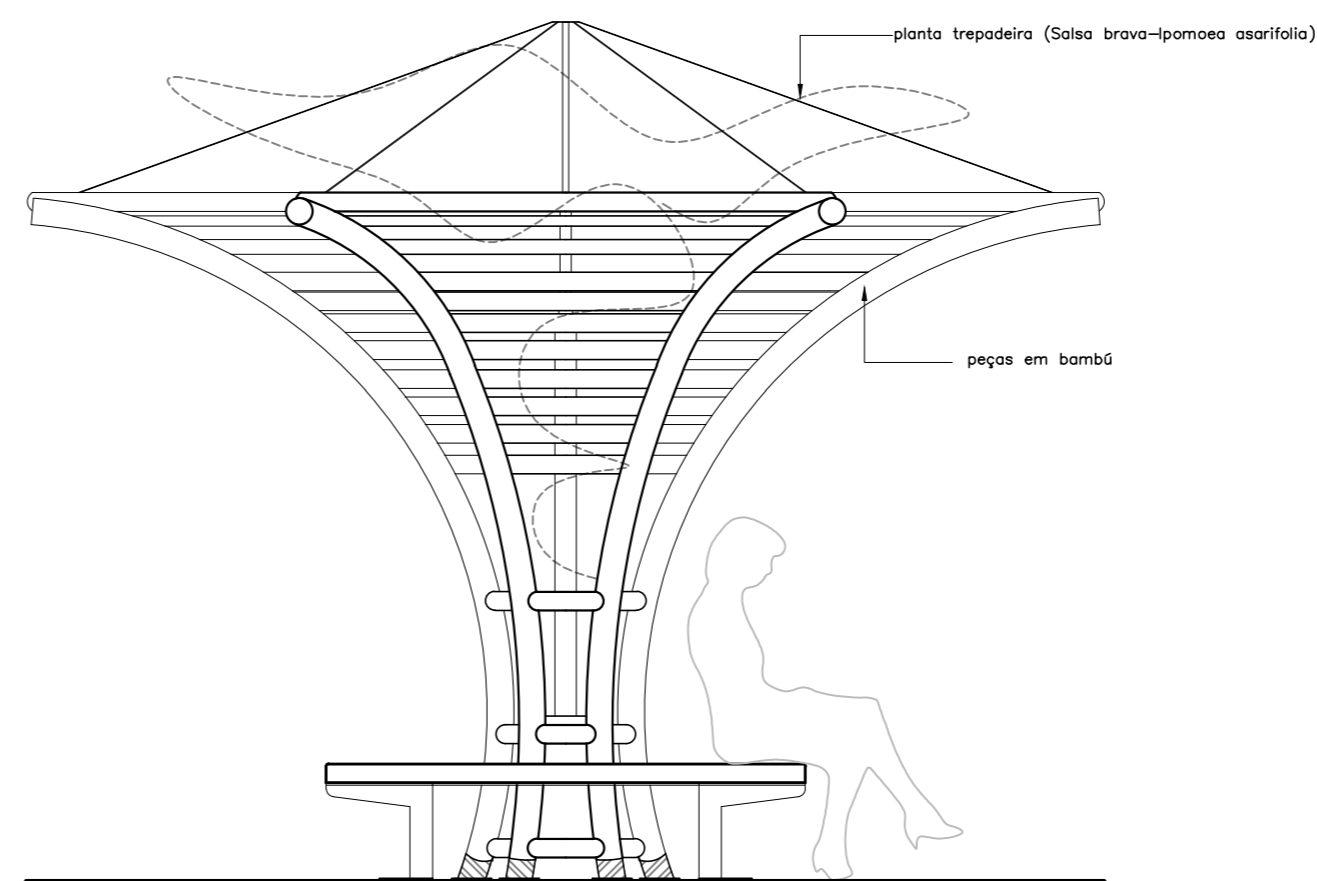
ELEVAÇÃO - PERGOLADO/BANCO CIRCULAR esc 1:20
