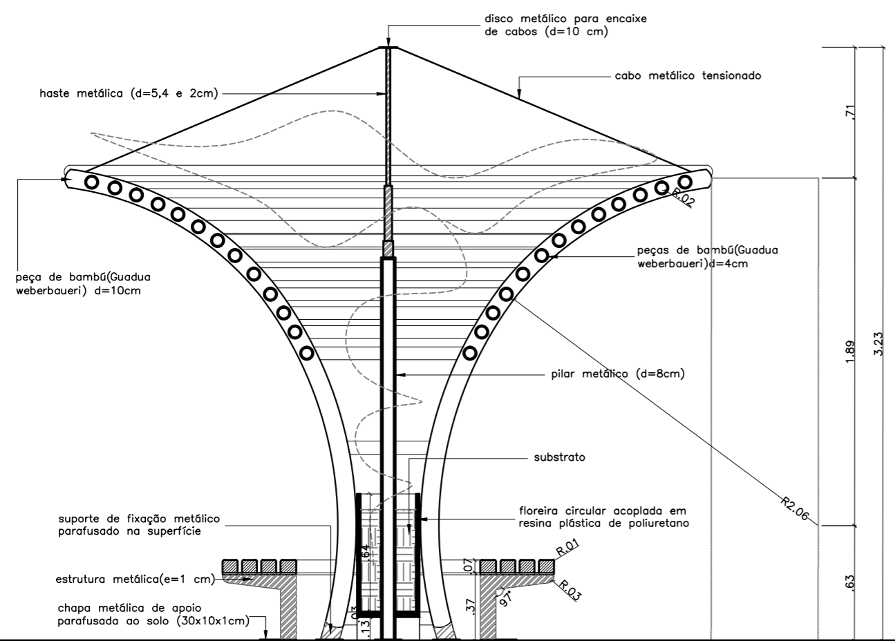
CORTE AA' - PERGOLADO/BANCO CIRCULAR esc 1:20
