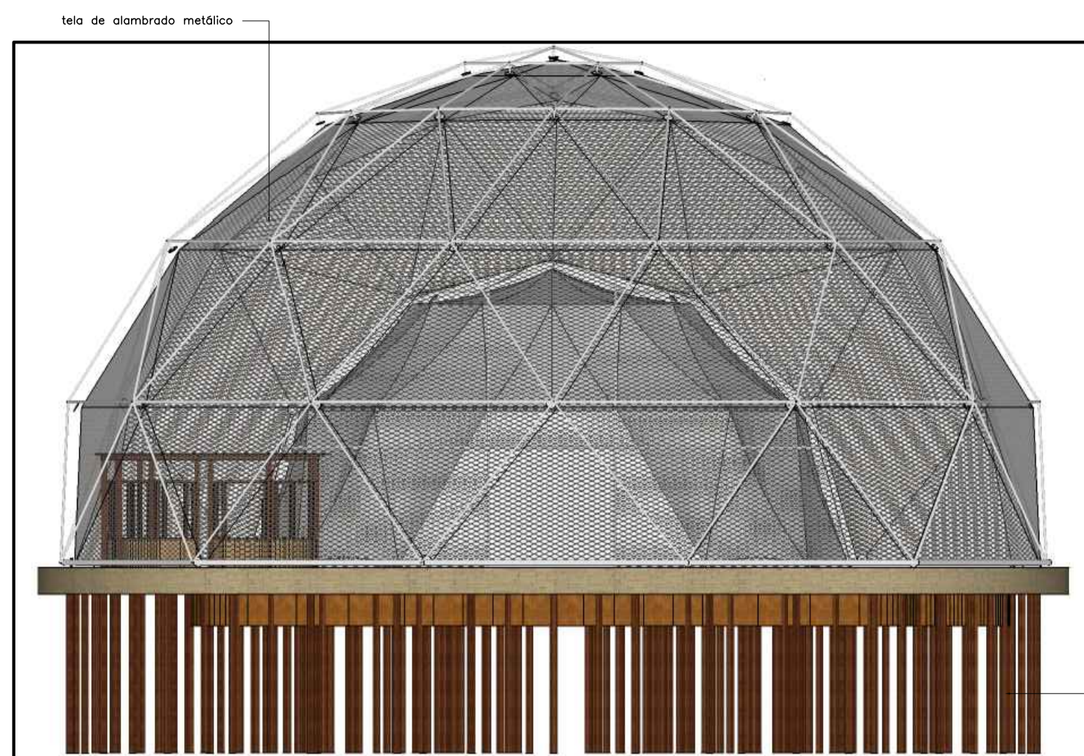
FACHADA POSTERIOR esc 1:100
