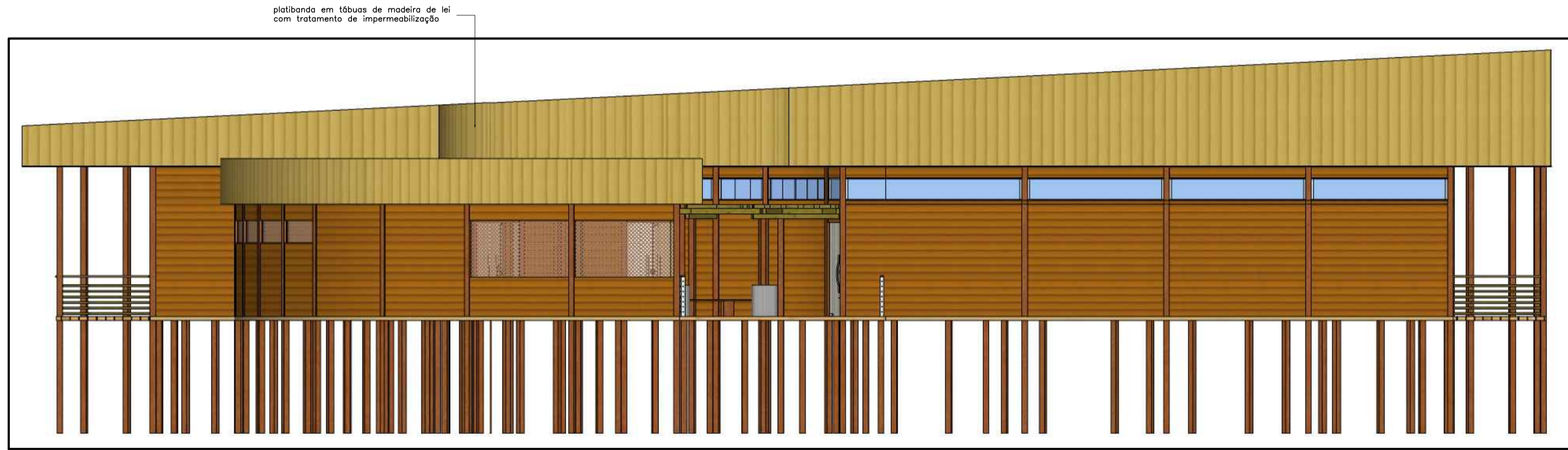
FACHADA FRONTAL esc 1:100
