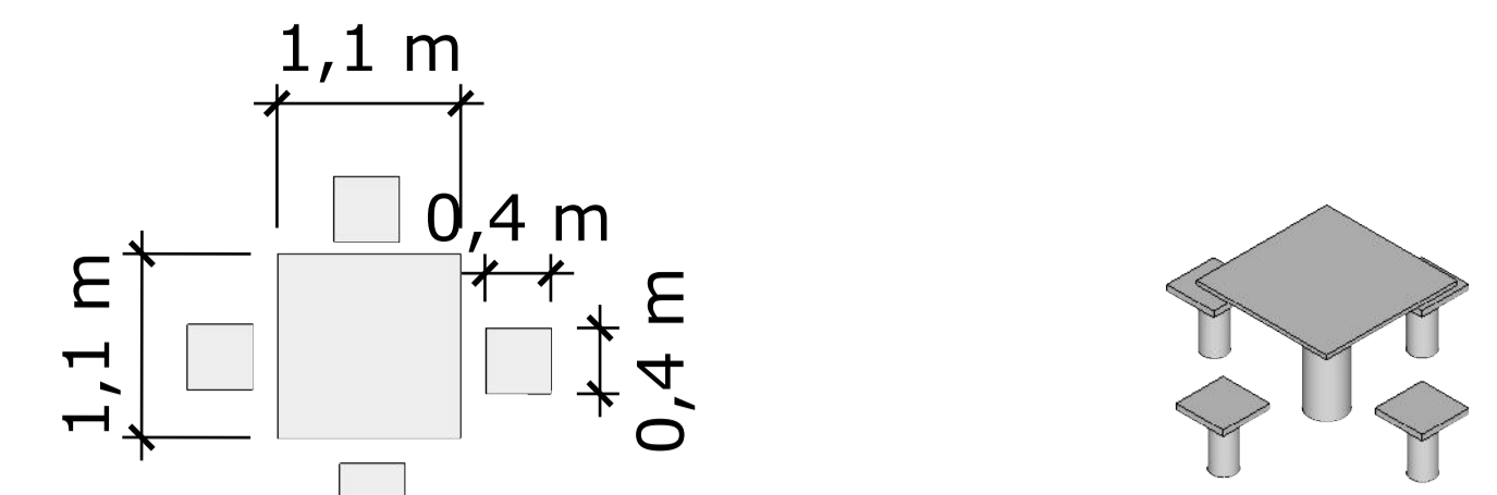
Vista Superior e Perspectiva Mesa em Concreto Det. 01 esc.: 1:50
