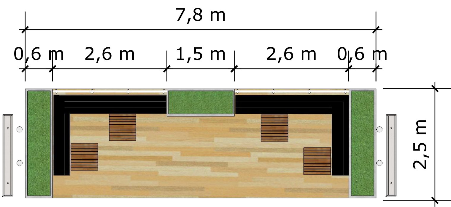
Det. Vista Superior Parklet Tipo 01 01 esc.: 1:50
