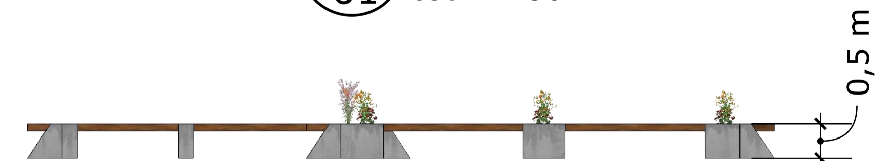
Vista Lateral Banco com Floreira Det. 01 esc.: 1:50
