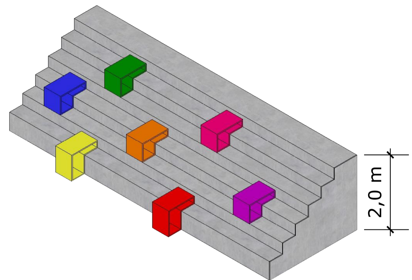
Det. Perspectiva Arquibancada 01 esc.: 1:50
