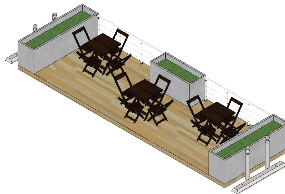
Det. Perspectiva Parklet Tipo 02 01 esc.: 1:50
