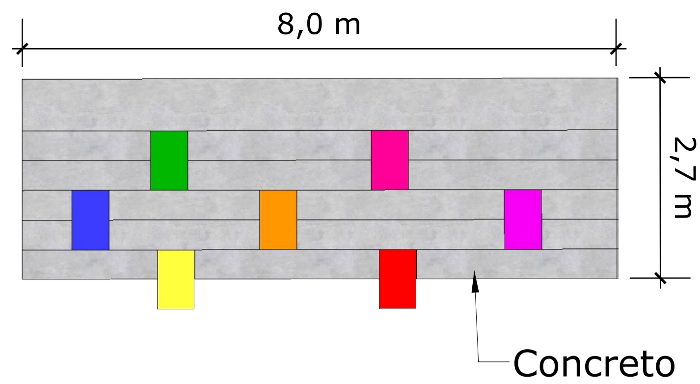
Det. Vista Superior Arquibancada 01 esc.: 1:50
