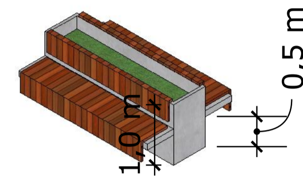
Perspectiva Banco com Canteiro Det. 01 esc.: 1:50
