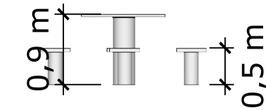
Det. Vista Lateral Mesa em Concreto 01 esc.: 1:50
