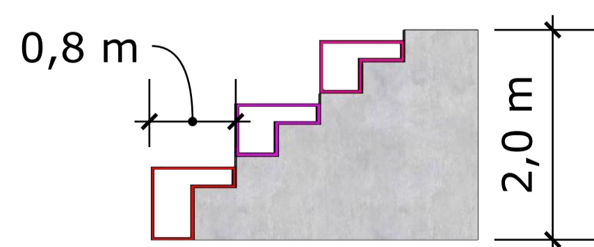
Det. Vista Lateral Arquibancada 01 esc.: 1:50
