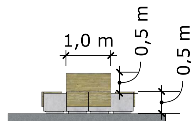
Vista Lateral Banco com Grelha de Escoamento Det. 01 esc.: 1:50
