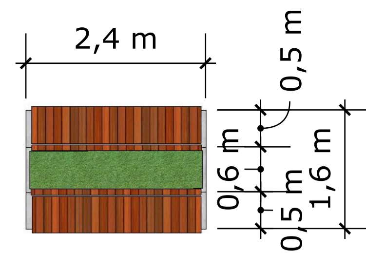
Vista Superior Banco com Canteiro Det. 01 esc.: 1:50
