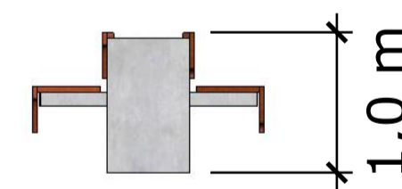
Vista Lateral Banco com Canteiro Det. 01 esc.: 1:50
