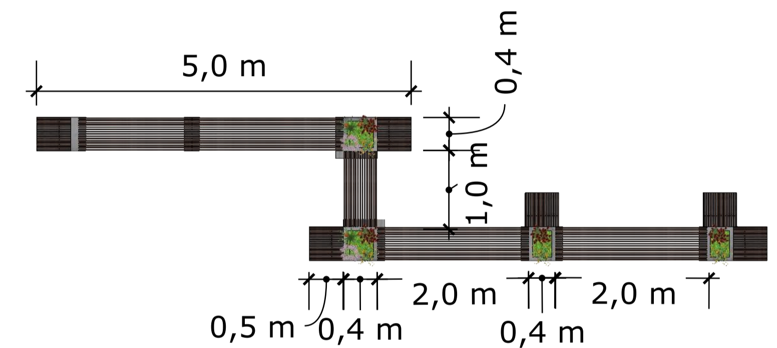
Det. Vista Lateral Mesa em Concreto 01 esc.: 1:50
