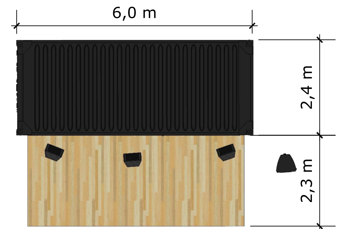
Det. Vista Superior Contêiner Palco 01 esc.: 1:50
