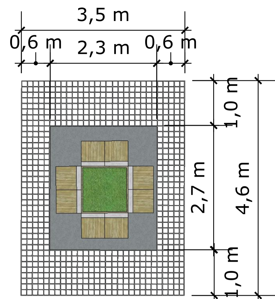
Vista Superior Banco com Grelha de Escoamento Det. 01 esc.: 1:50
