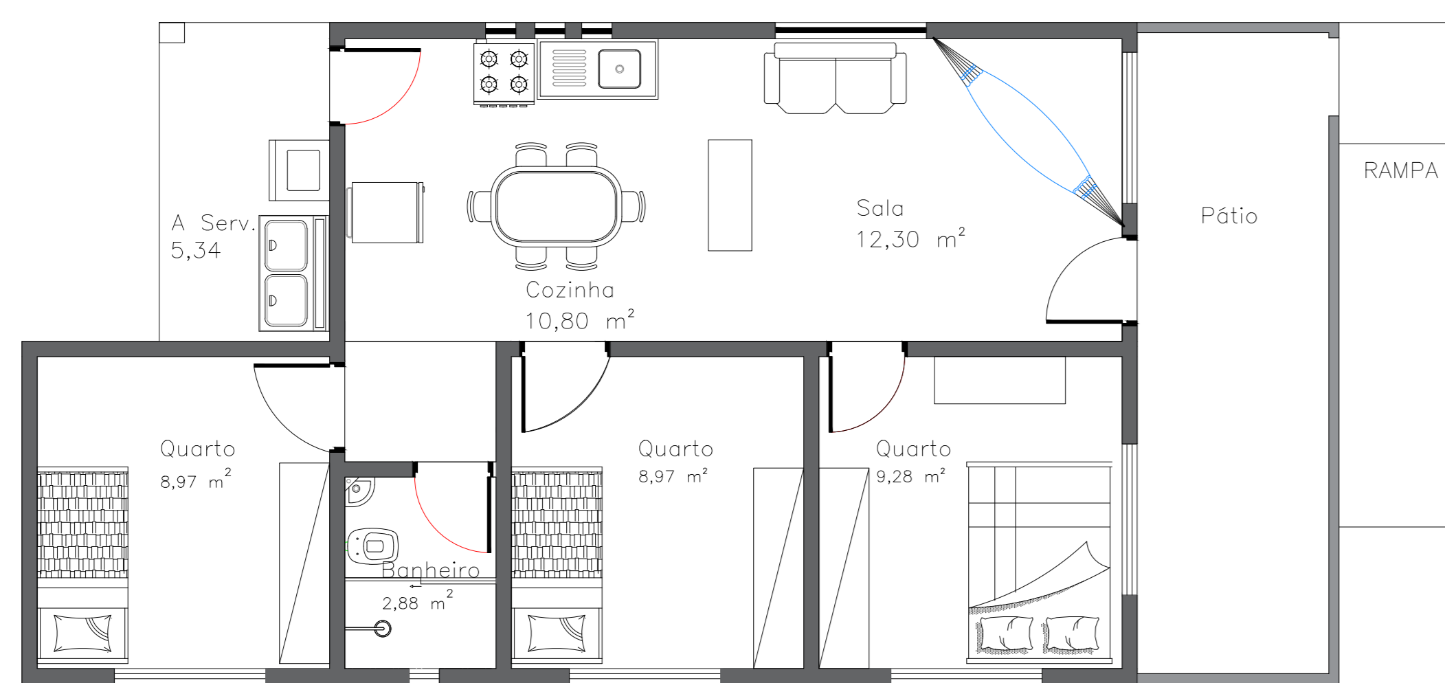
PLANTA BAIXA HABITAÇÃO TIPO 2 ESC. 1:50
