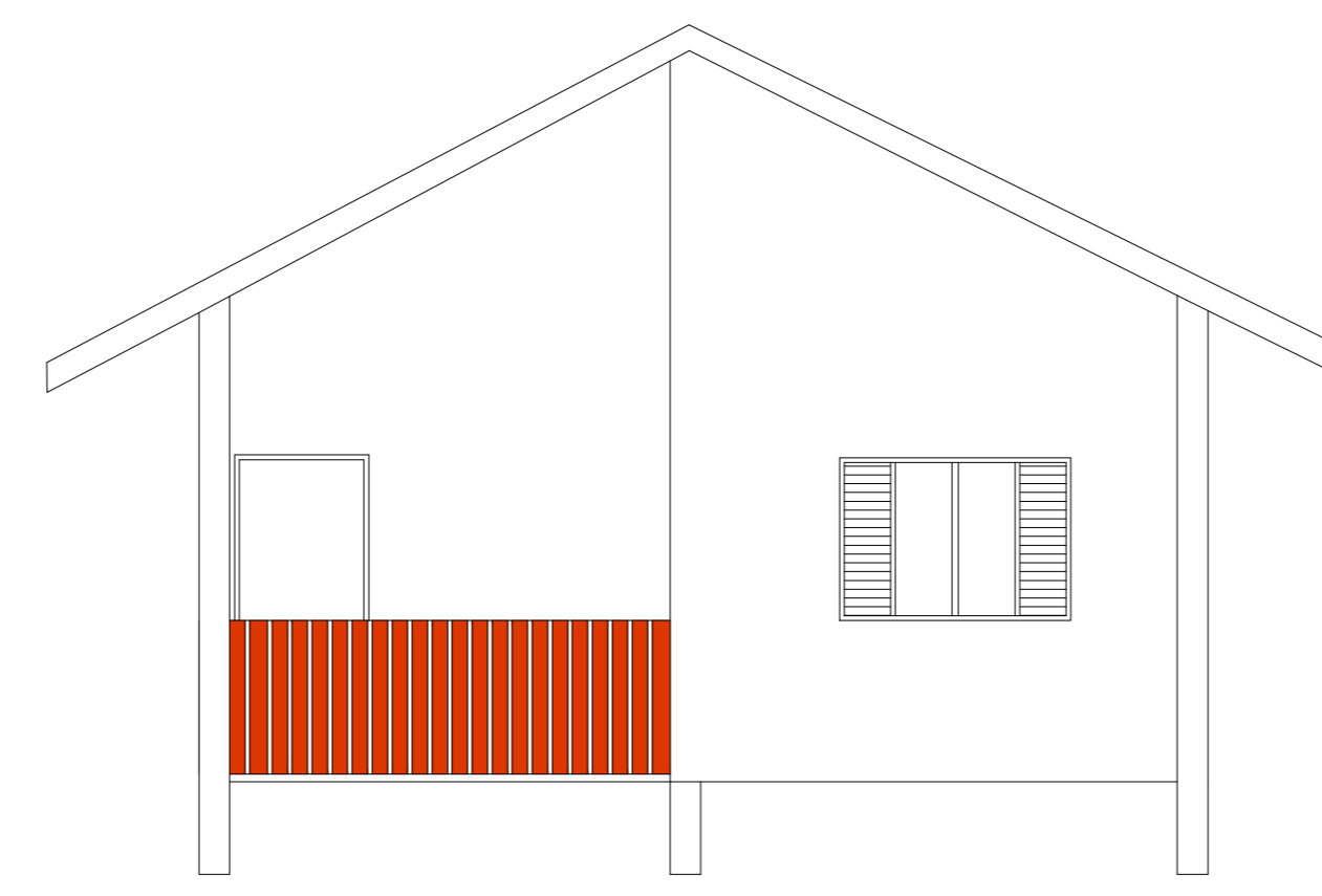
FACHADA POSTERIOR ESC. 1:50
