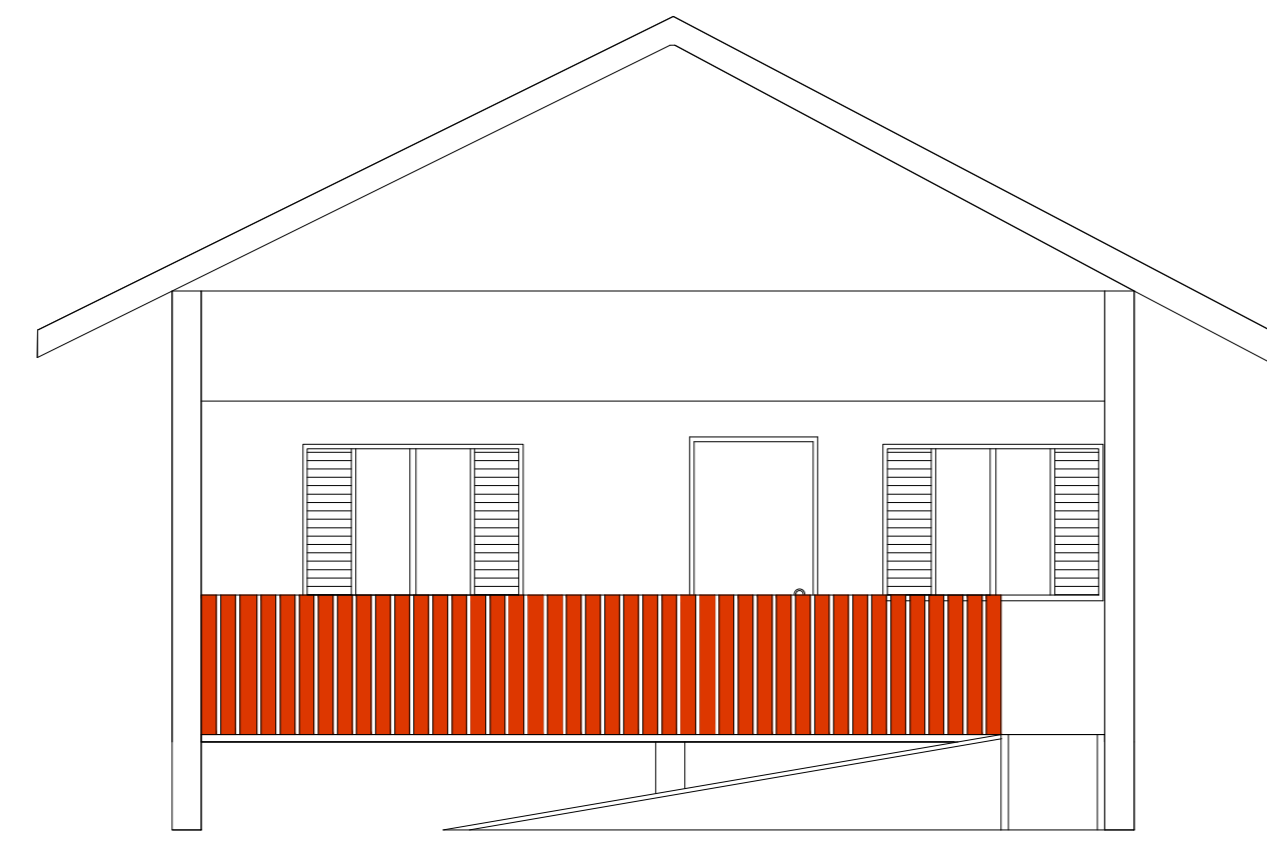
FACHADA FRONTAL ESC.1:50
