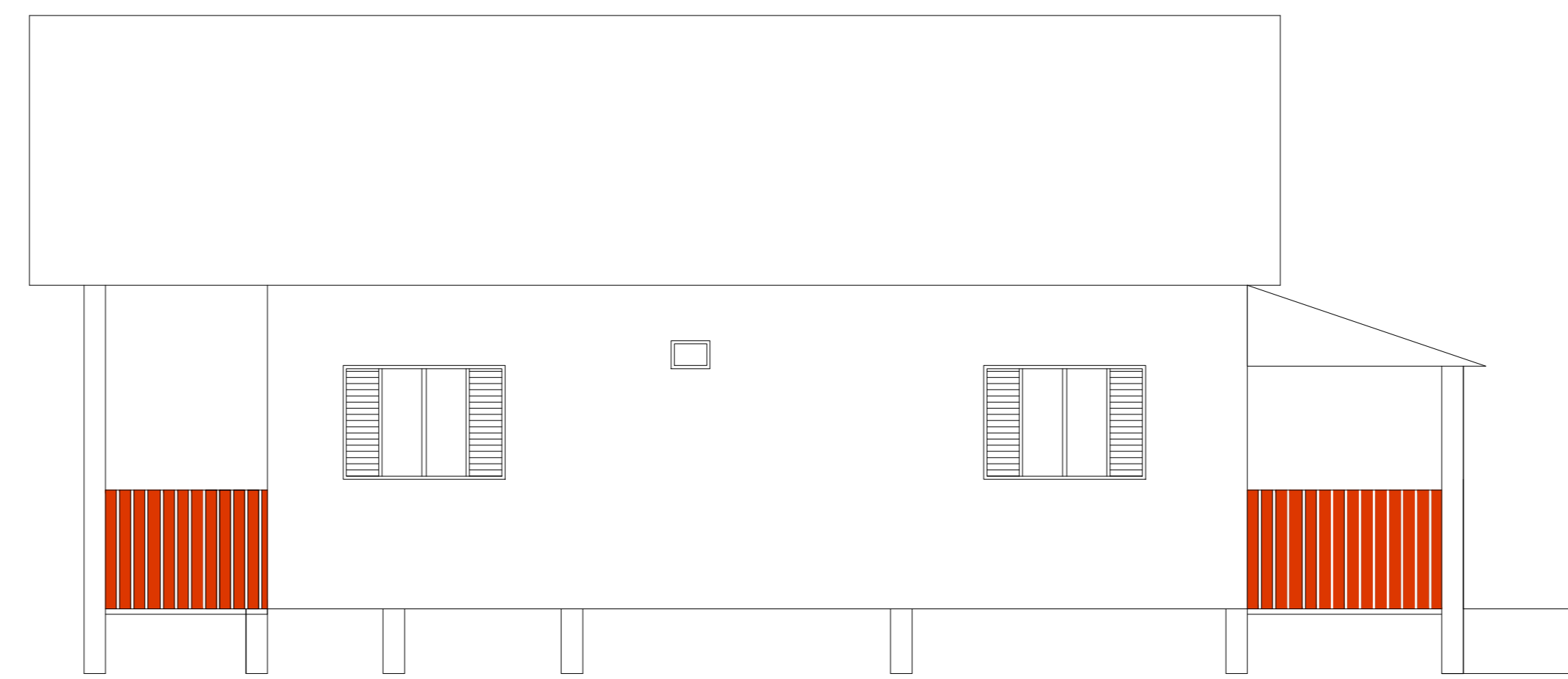
FACHADA LATERAL SUL ESC.1:50
