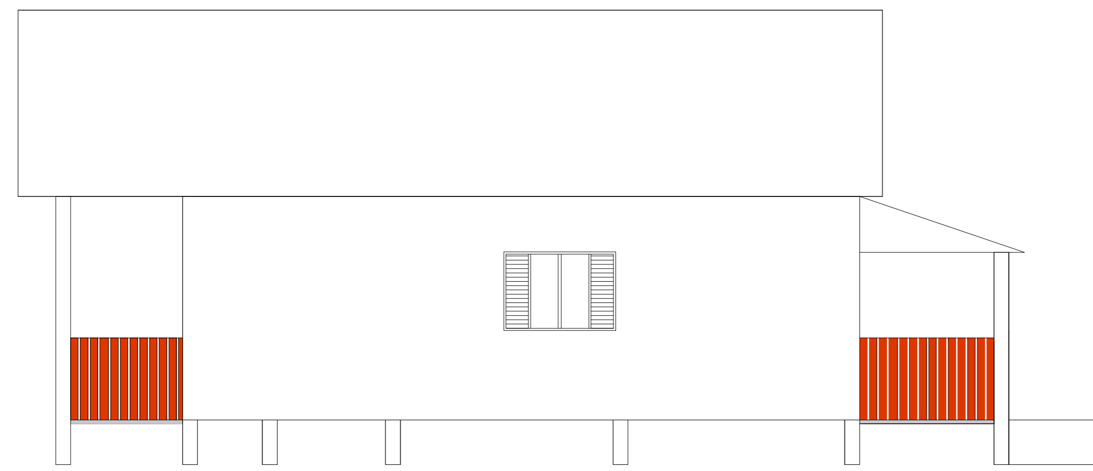
FACHADA LATERAL NORTE ESC.1:50
