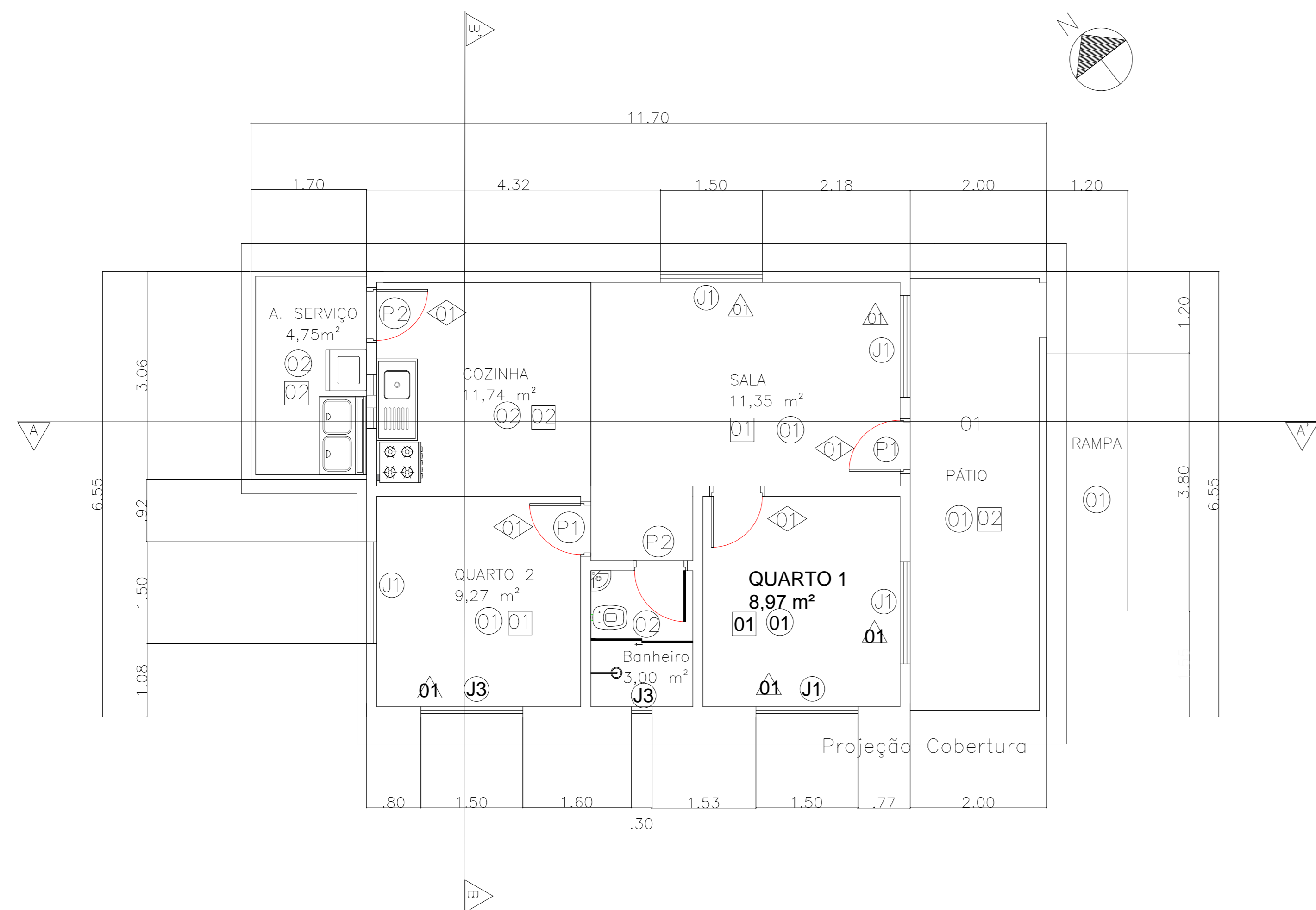
PLANTA BAIXA HABITAÇÃO TIPO 1 ESC. 1:50
