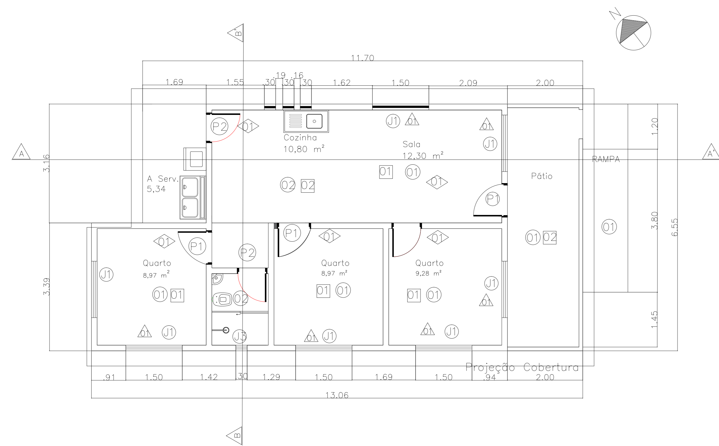
PLANTA BAIXA HABITAÇÃO TIPO 2 ESC. 1:50
