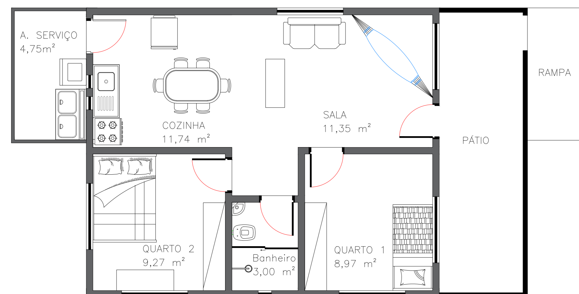
PLANTA LAYOUT HABITAÇÃO TIPO 1 ESC. 1:50
