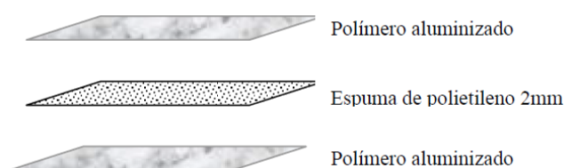
Figura 126 – Manta de alumínio (subcobertura)
