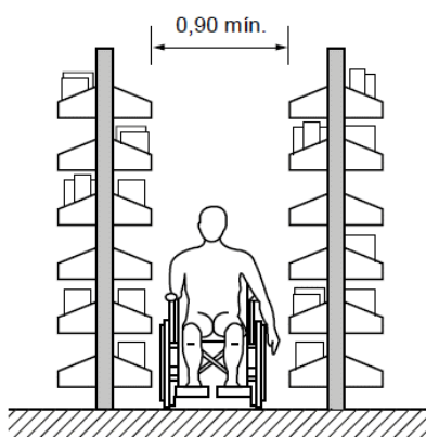
Figura 39 - Largura entre estantes em bibliotecas – exemplo – vista frontal.
