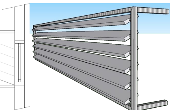
Figura 157 – Perspectiva brise horizontal infinito – fixo – fachada oeste.
