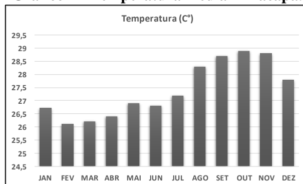
Gráfico 2 - Temperatura média – Macapá.
