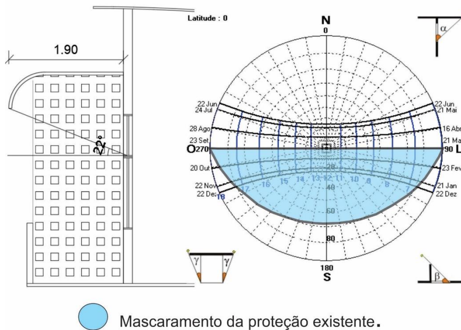
Figura 125 – Mascaramento da fachada sul (balancim)
