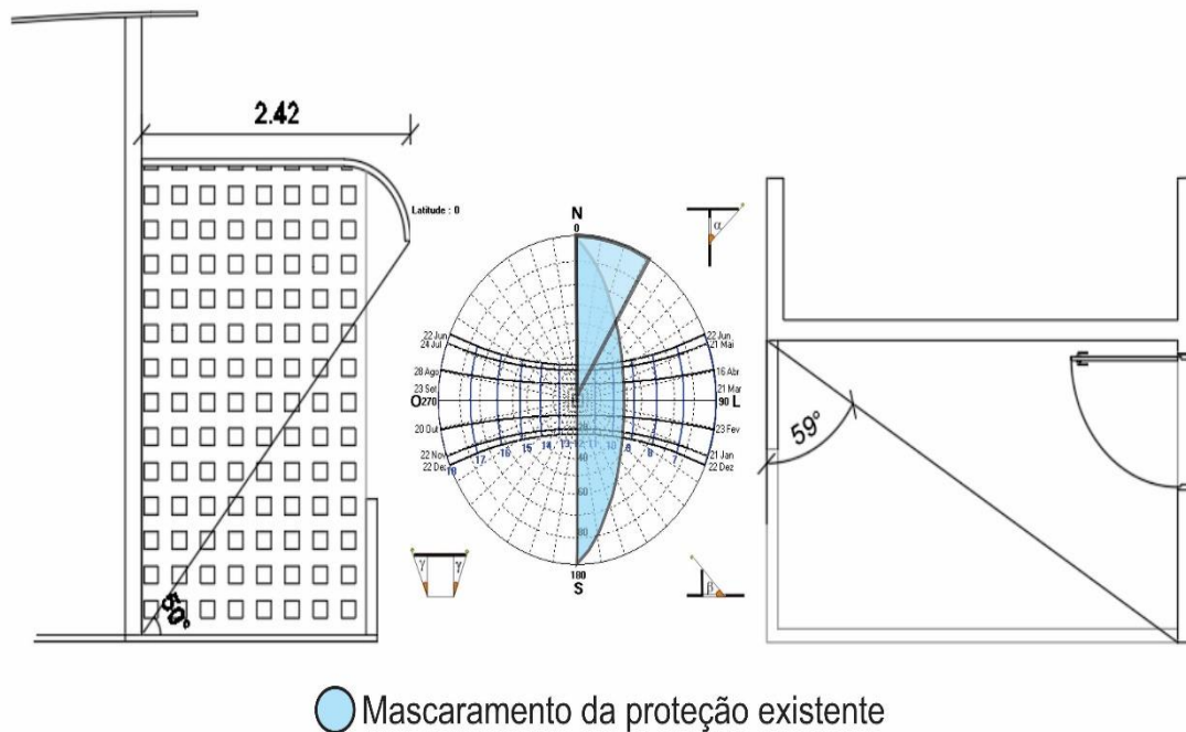
Figura 127 – Mascaramento da fachada leste
