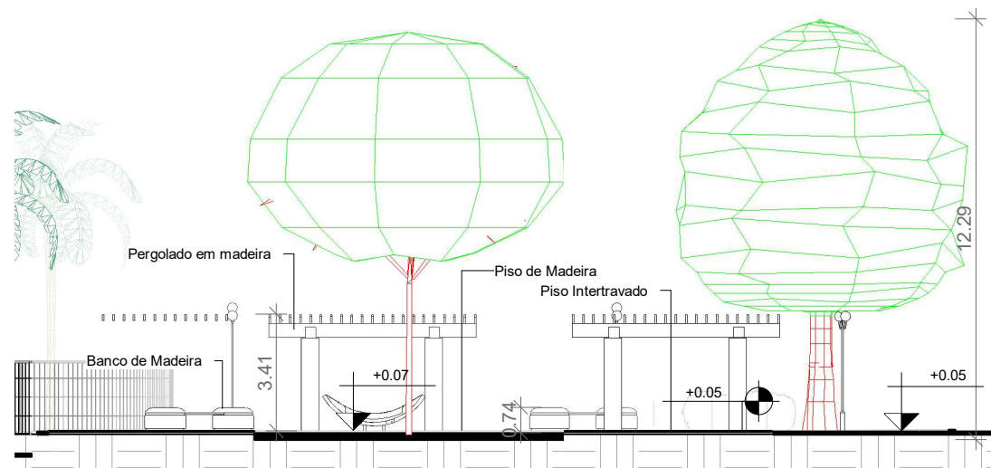
6 CORTE REDARIO ESCALA 1 : 200
