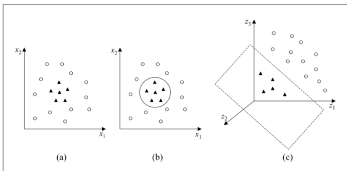
Figura 9 – Função Kernel.
