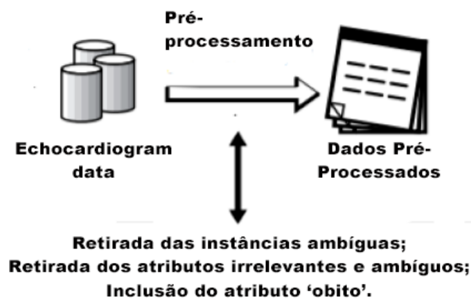
Figura 12 – Pré-processamento
