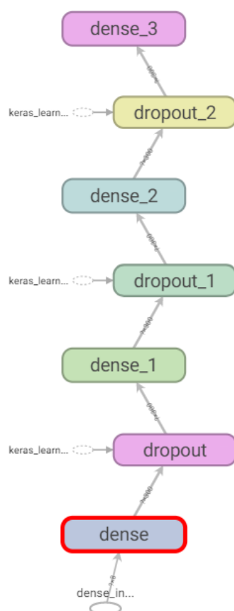
Figura 10 – Gráfico conceitual gerado pelo TensorFlow
