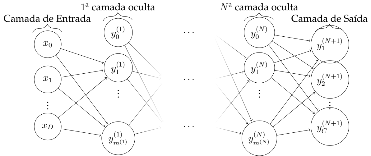
Figura 2 – Exemplo de uma rede neural Multilayer Perceptron
