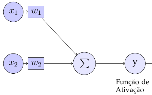
Figura 1 – Exemplo de arquitetura Perceptron
