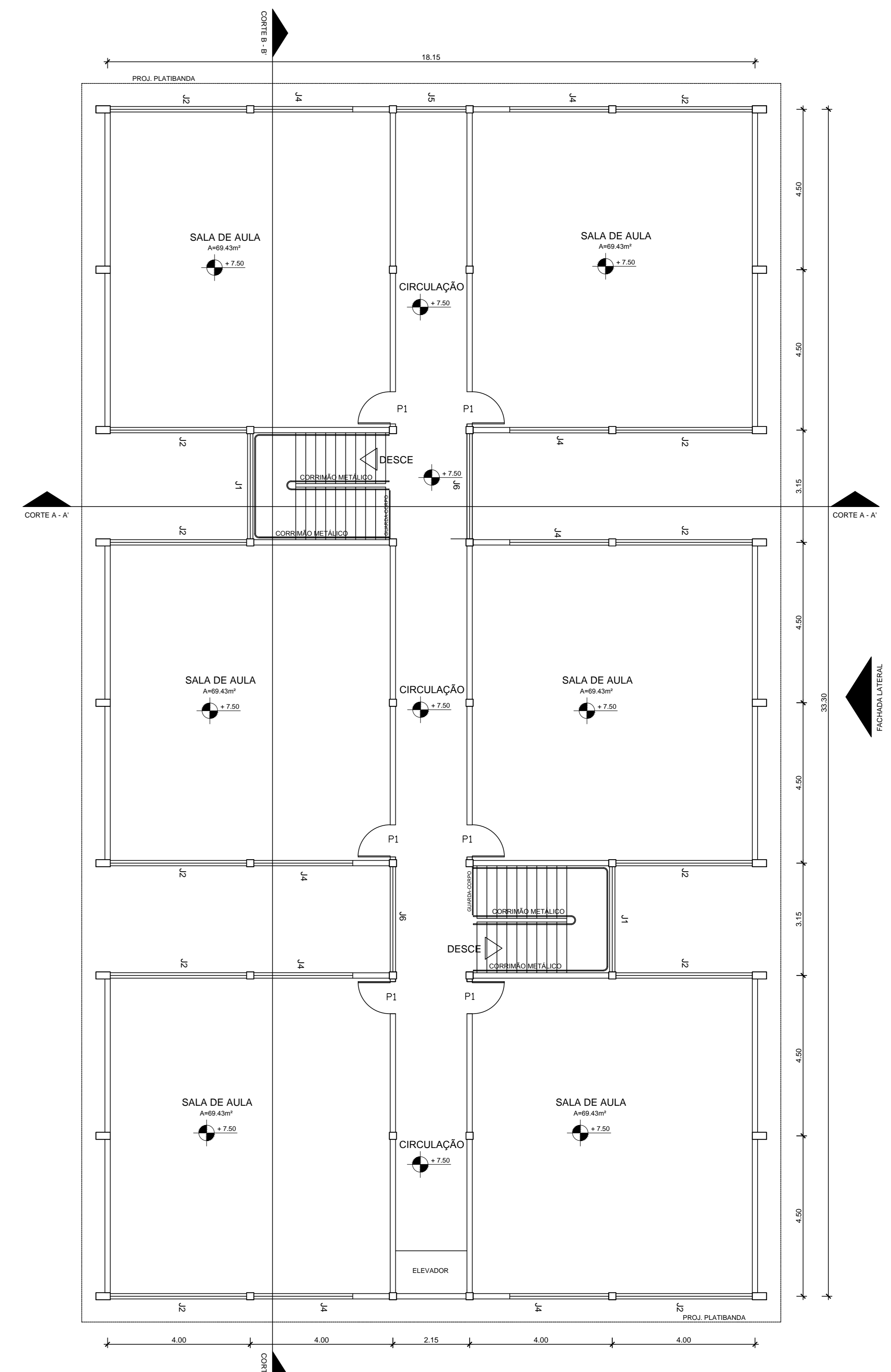
BLOCO B 3º PAVIMENTO (Área: 540,18m²)
