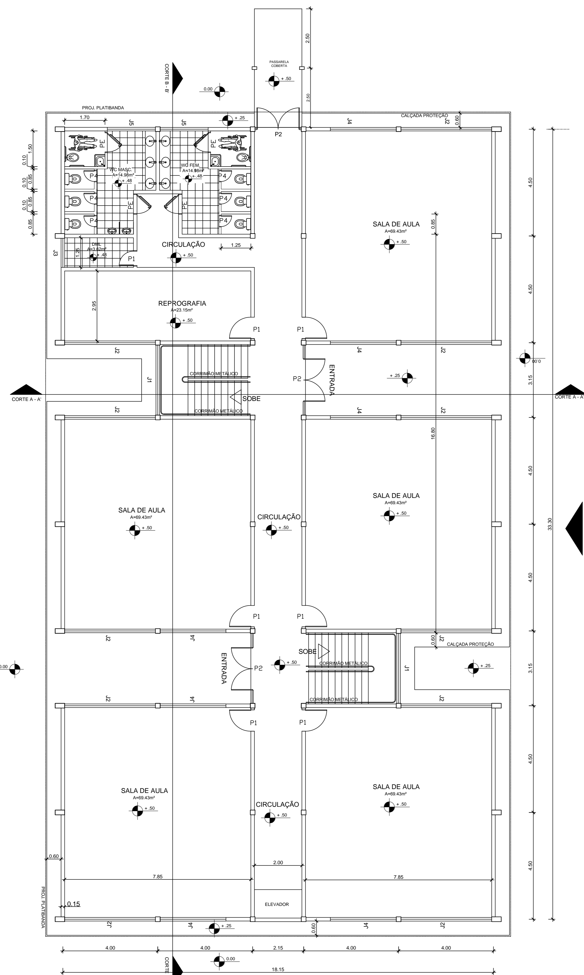
BLOCO B PAVIMENTO TÉRREO (Área: 540,18m²)
