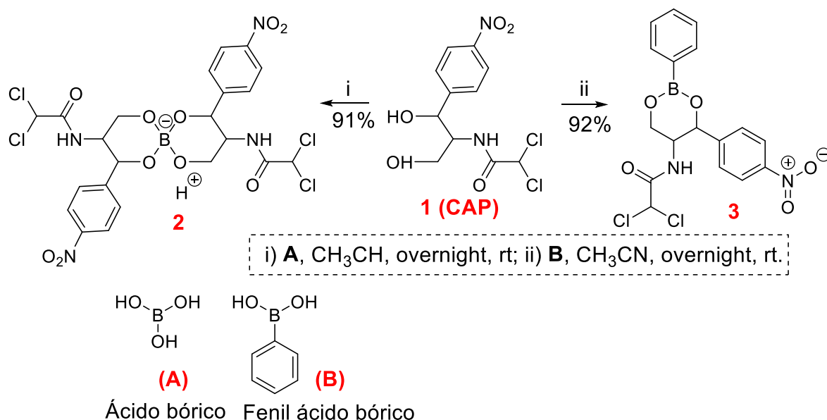
Esquema 3. Síntese de cloranfenicol borato e fenilboronato .
