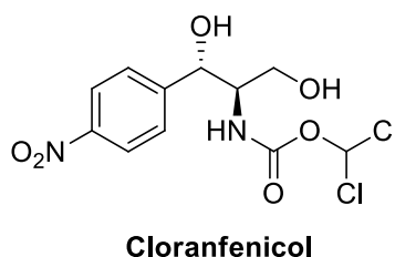
Figura 1. Estrutura química do cloranfenicol.
