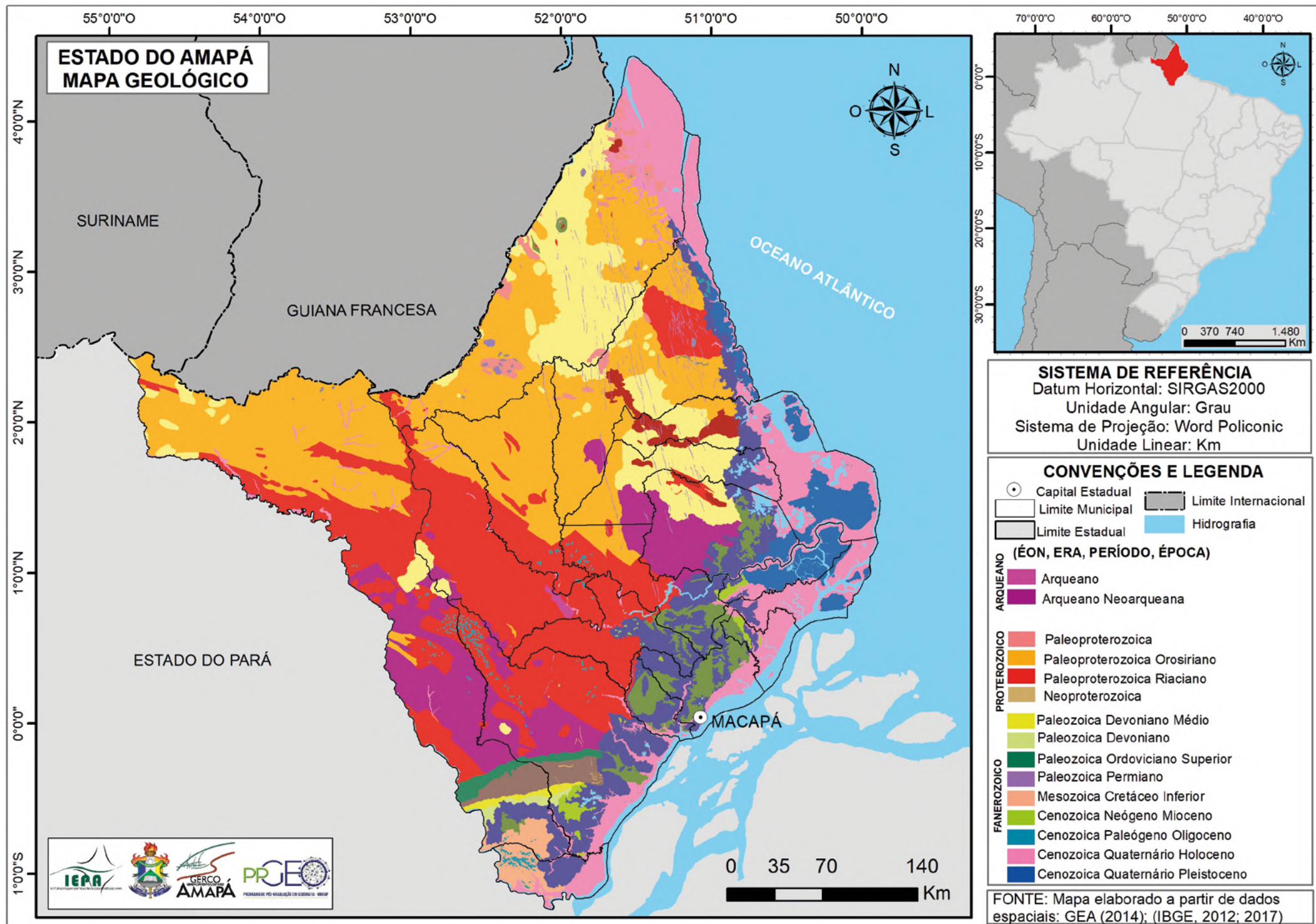
Mapa 23: GEOLOGIA DO ESTADO DO AMAPÁ
