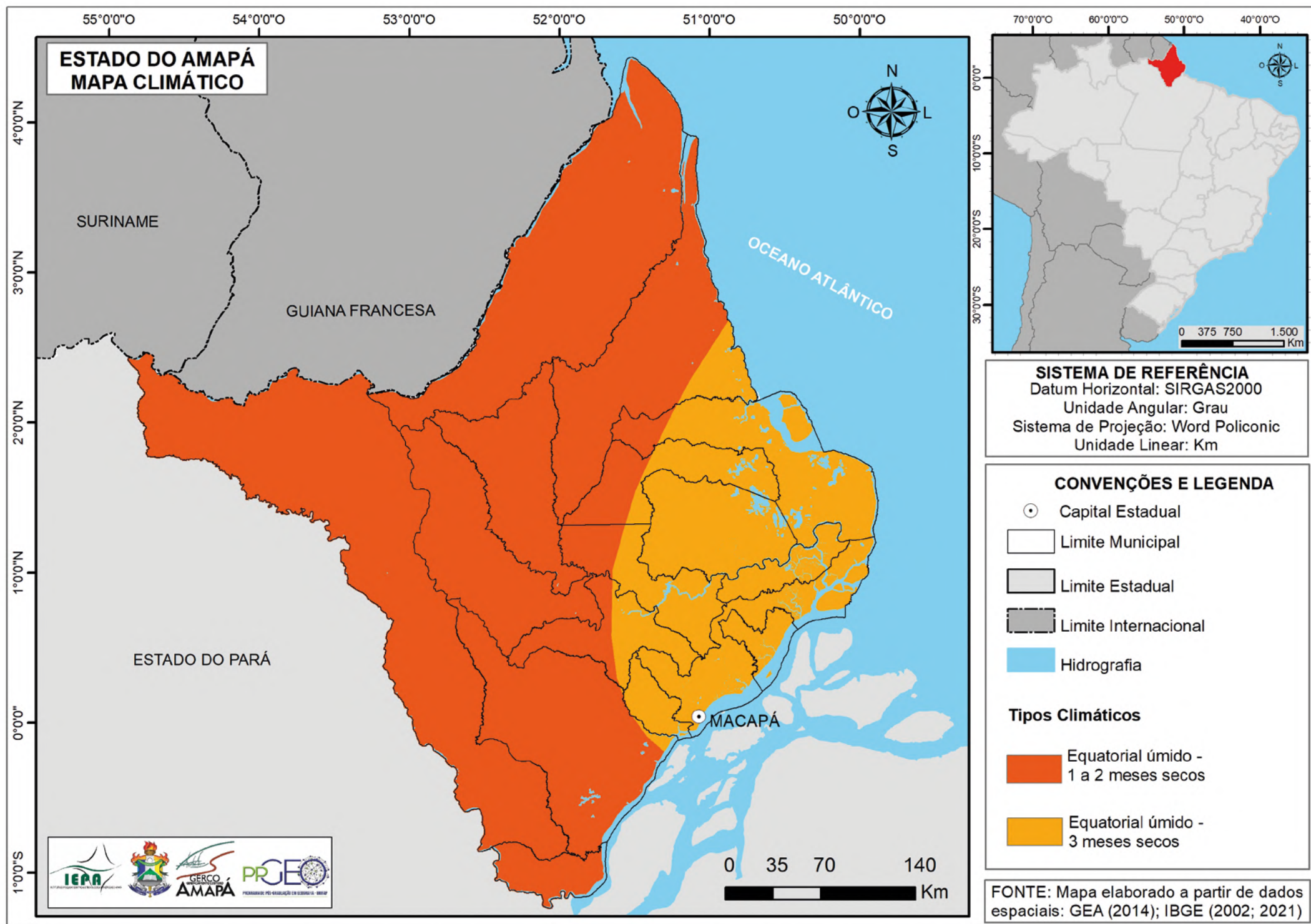
Mapa 21: CLIMAS DO ESTADO DO AMAPÁ
