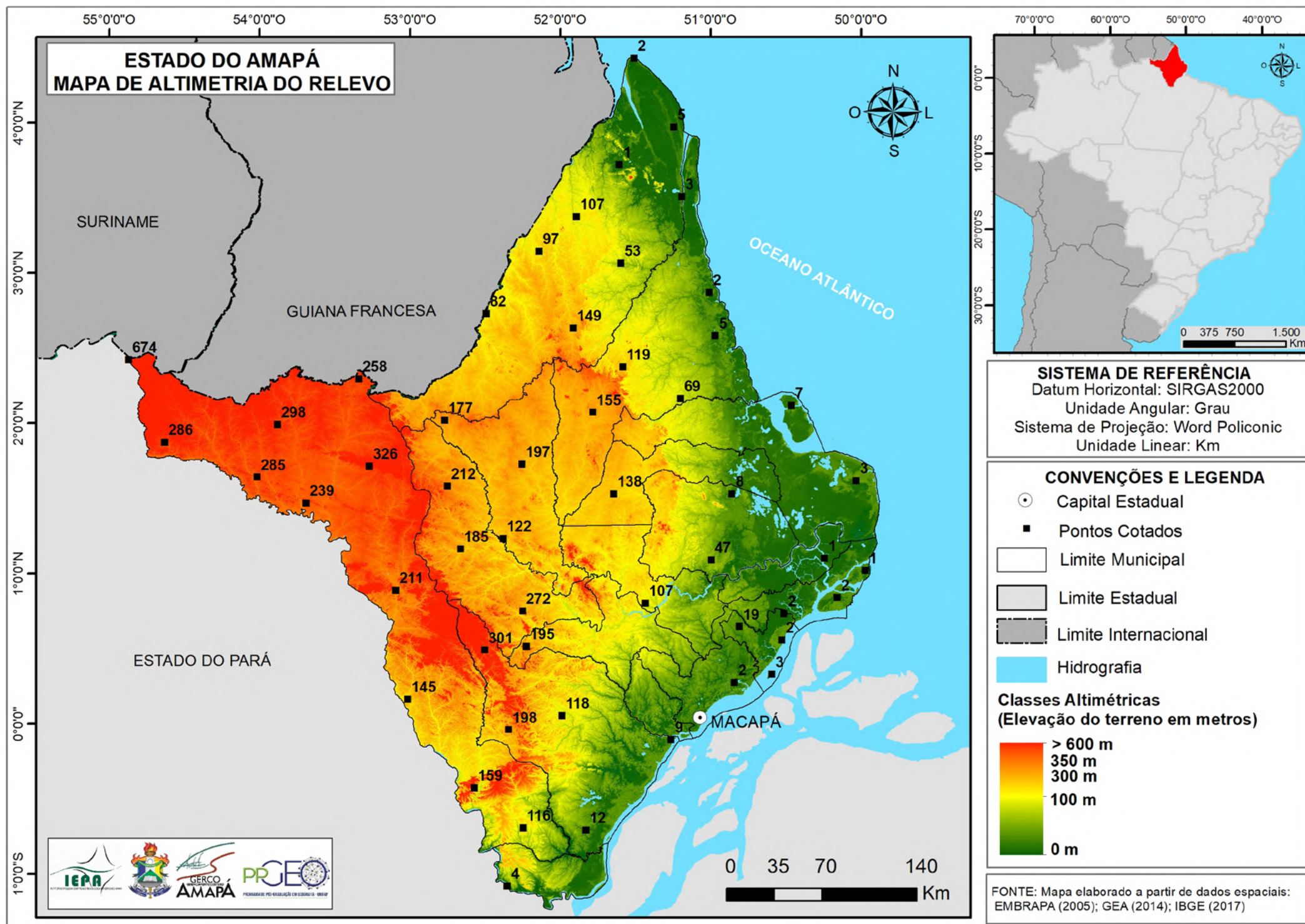
Mapa 25: ALTIMETRIA DO RELEVO DO ESTADO DO AMAPÁ
