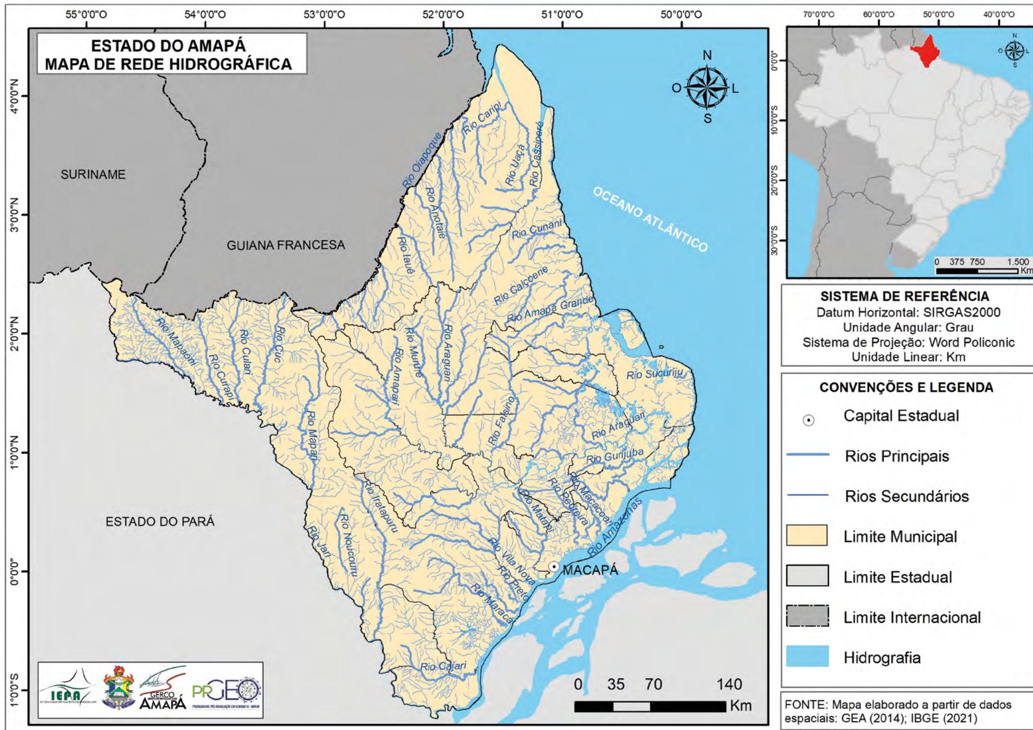
Mapa 26: REDE HIDROGRÁFICA DO ESTADO DO AMAPÁ
